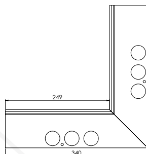
Kút – PRIAMY/FLEXI Materiál: Al
