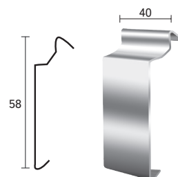
Spojka – PRIAMY/FLEXI Materiál: Al
